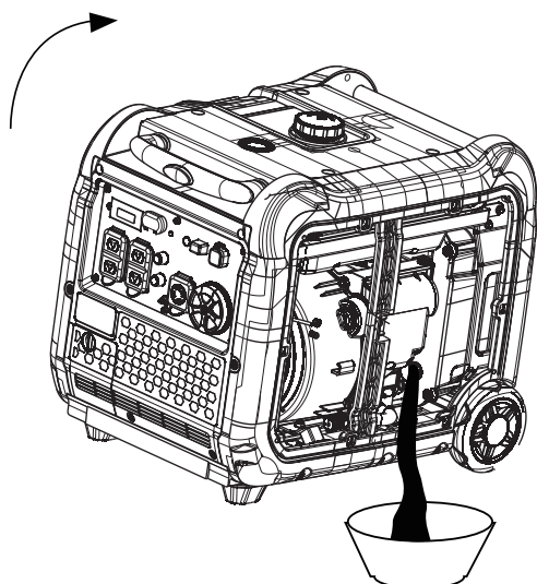
Figure 10: Inclinez délicatement l'onduleur pour que l'huile s'écoule dans le bac à huile.
