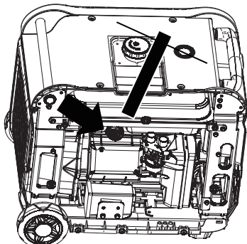
Abbildung 16: Entfernen der Zündkerze mit dem Steckschlüssel
