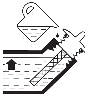
Abbildung 4: Richtiger Motorölstand
