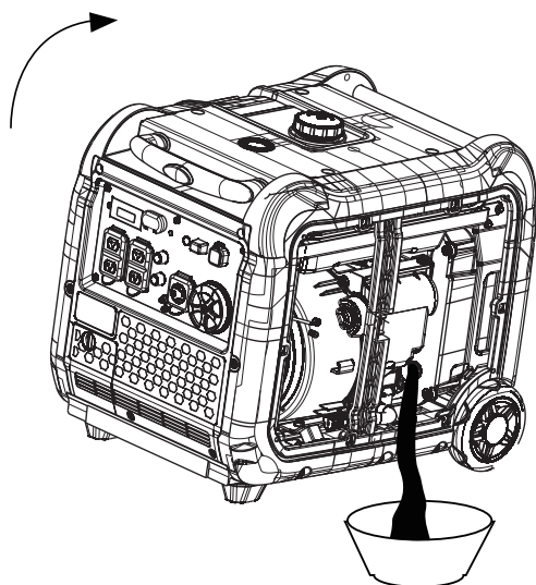
Abbildung 10: Kippen Sie den Wechselrichter vorsichtig, damit das Öl in die Ölwanne fließt.
