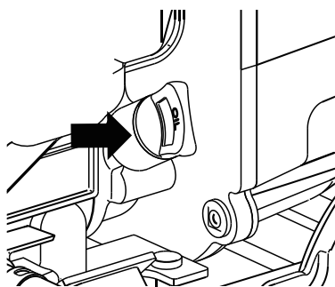
Abbildung 2: Öleinfüll-/Ablassschraube
